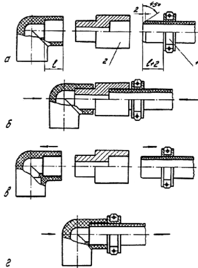
Рис. 9. Последовательность процесса контактной сварки внастроб труб и соединительных деталей из ПВД: а - центровка, закрепление в зажимах сварочного устройства концов свариваемых труб и деталей и установка ограничительного хомута 1; б - установка дорна нагретого инструмента 2 в раструбе и гладкого конца трубы в гильзе; в - нагрев (оплавление) свариваемых концов, одновременно снятие их с дорна и гильзы; г - соединение концов с выдержкой до затвердевания сплавленного материала
