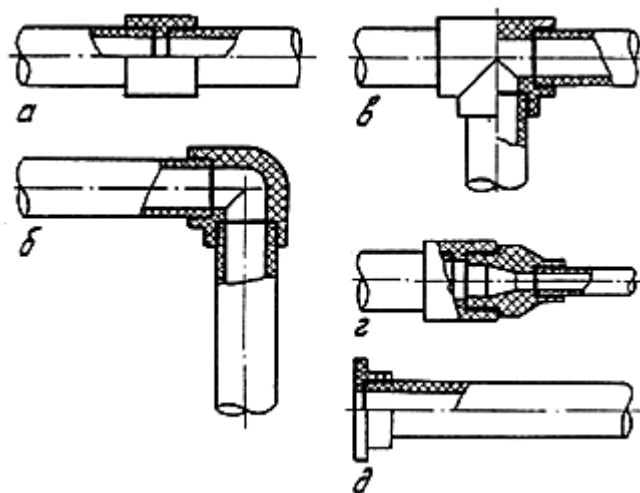
Рис. 6. Сварные раструбно-стыковые соединения труб и соединительных деталей из ПВД:
