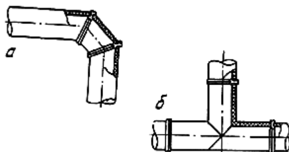
Рис. 5. Сварные стыковые соединения труб со сварными соединительными деталями: а - труб с угольником 90°; б - труб с тройником
