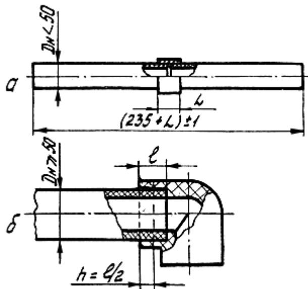
Рис. 2. Образцы для испытаний сварных раструбных соединений: а - на сдвиг растяжением; б - на сдвиг сжатием с вырезкой кольцевого образца; L - длина муфты; l - глубина раструба; h - высота кольцевого образца
