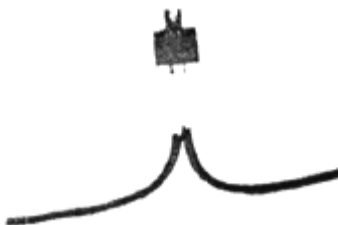
Рис. 11. Подготовленные к огарке жилы кабеля с термитным патроном марки АС
