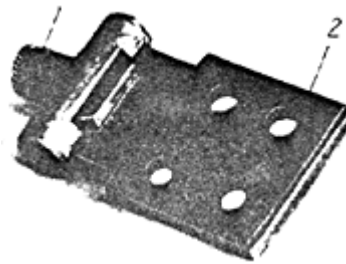
Рис.25. Оконцованный алюминиевый кабель с применением полуформ, изготовленных на базе набора НГО: 1 - кабель; 2 - контактная пластина
