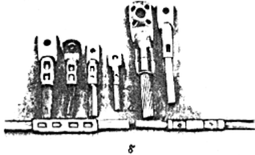
Рис. 27. Образцы оконцевания алюминиевых жил кабелей, выполненные способом опрессовки: а - оконцованные жилы кабеля; б - соединенные жилы кабеля
