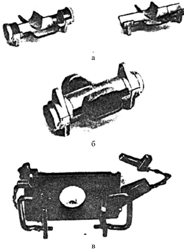
Рис. 22. Сварочные полуформы: а - сварочные полуформы в разобранном виде; б - сварочные полуформы в собранном виде; в - зажимные устройства полуформы
