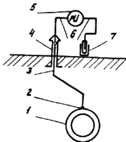
Рис. 31. Схема измерений разности потенциалов "труба -земля":
