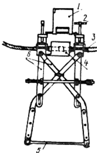
Рис.10. Сварочные клещи типа АТСП-50-185:
