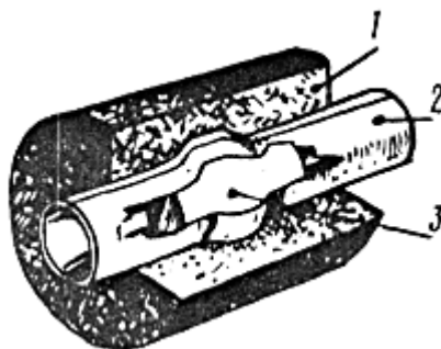
Рис .9. Термитный патрон марки АС для сварки жил проводов и кабелей:
